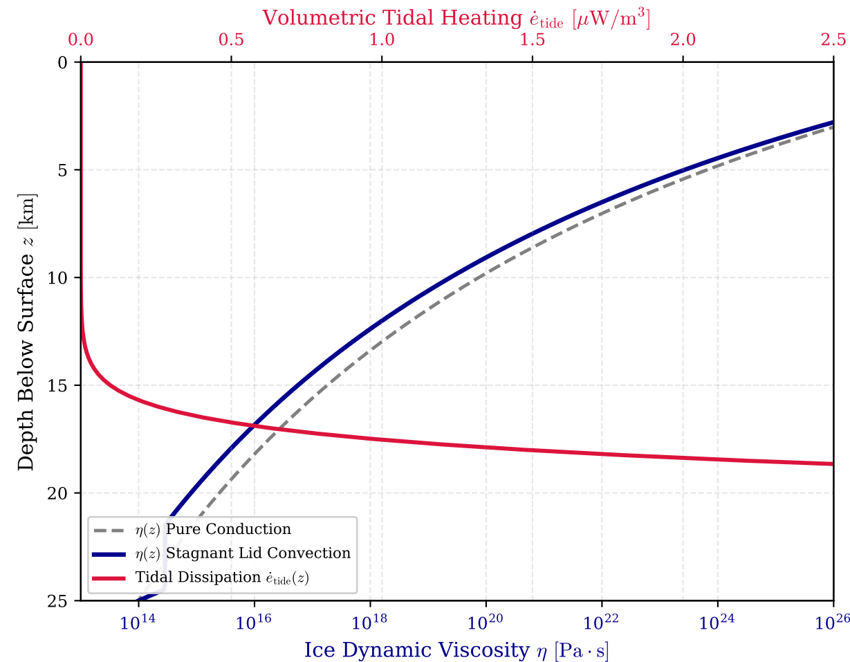
(d) Rheology & Volumetric Tidal Heating
