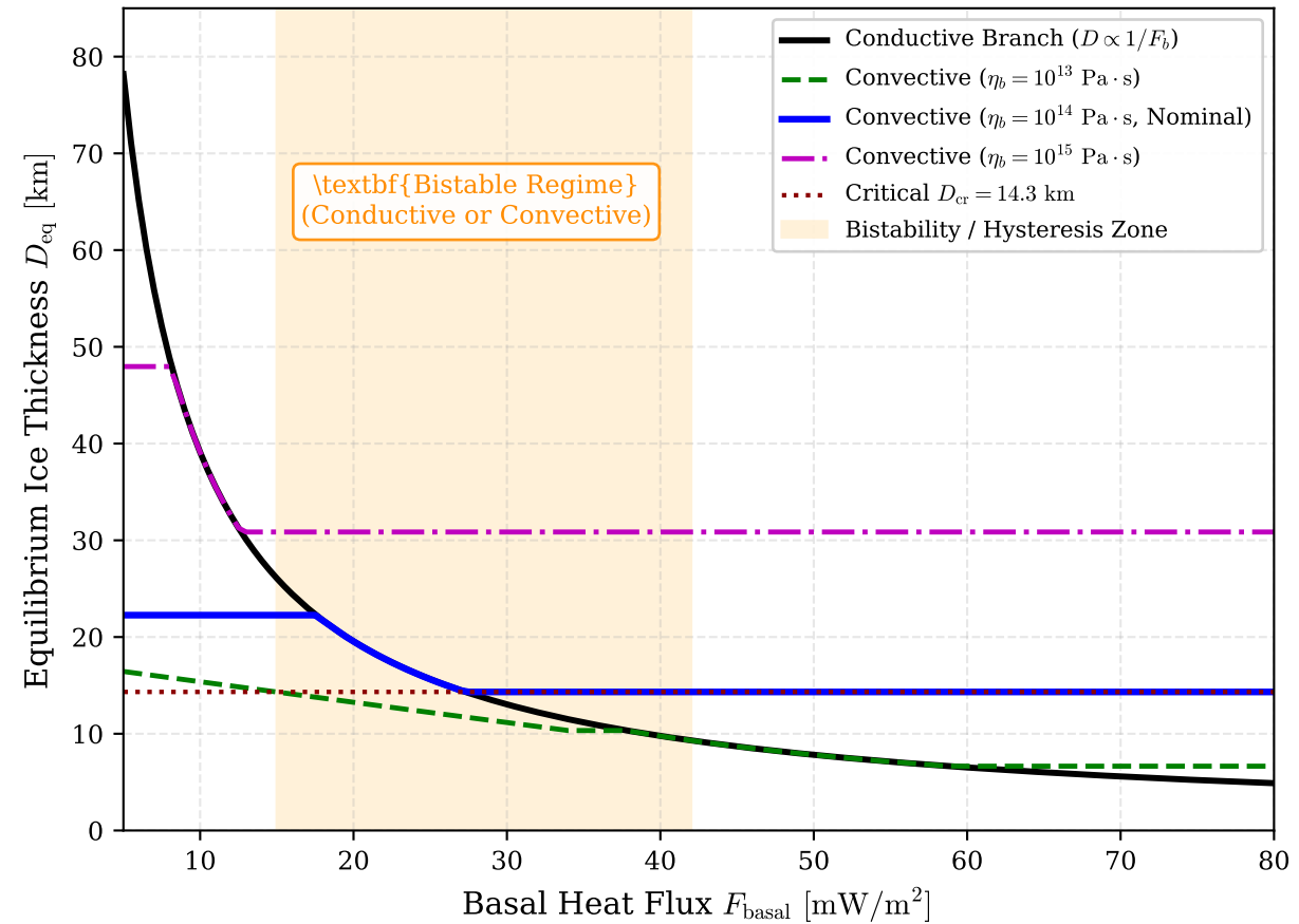
(d) Rheology & Volumetric Tidal Heating
