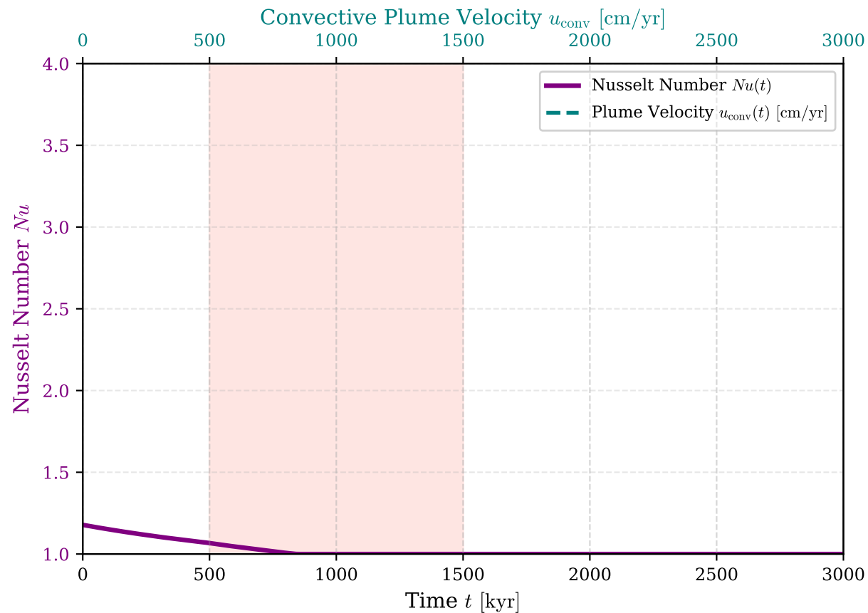
(d) Convective Vigour & Upwelling Plume Dynamics
