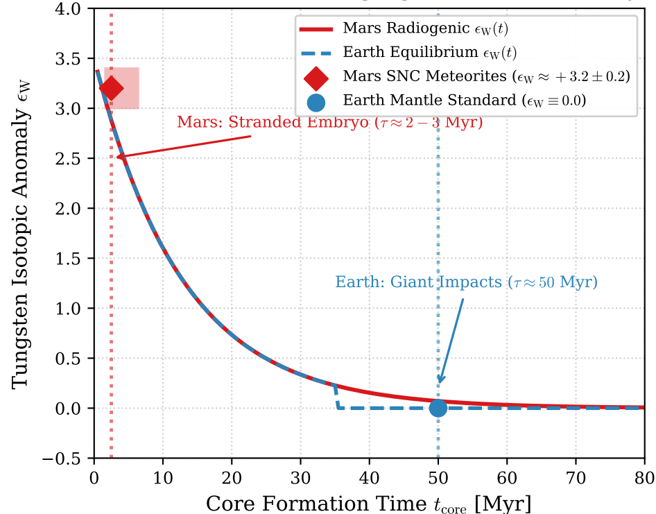
(d) ^{182}\text{Hf} - ^{182}\text{W} Core Segregation Chronometry
