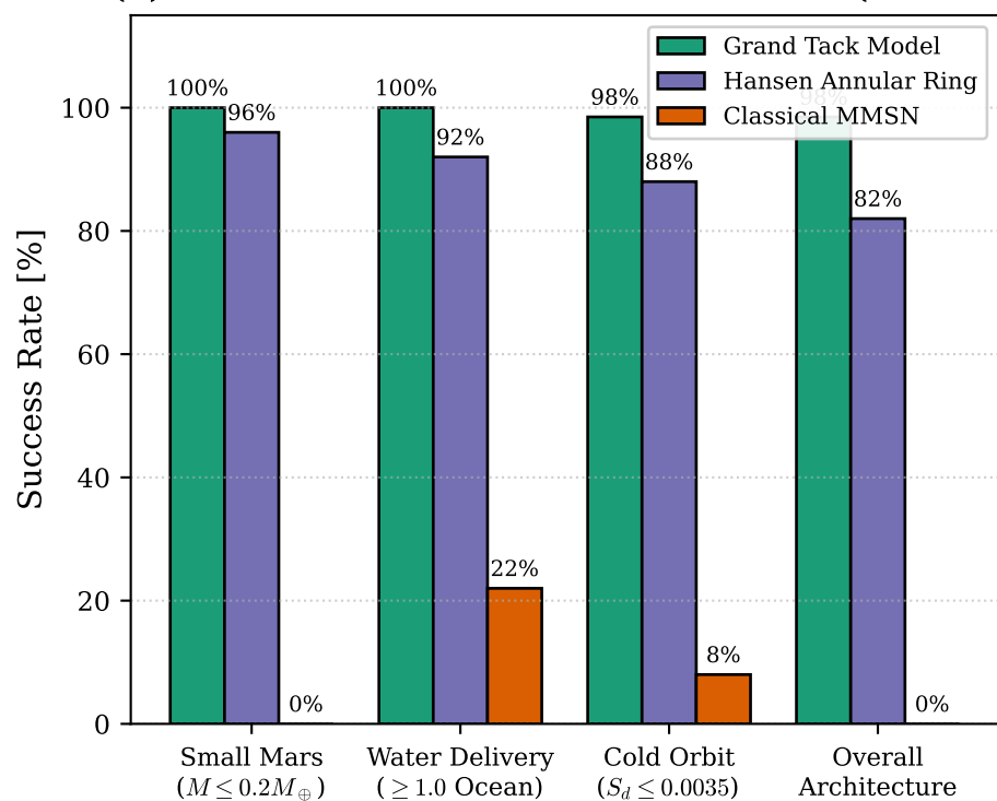
(d) Statistical Ensemble Success Rates ( N = 1000 )
