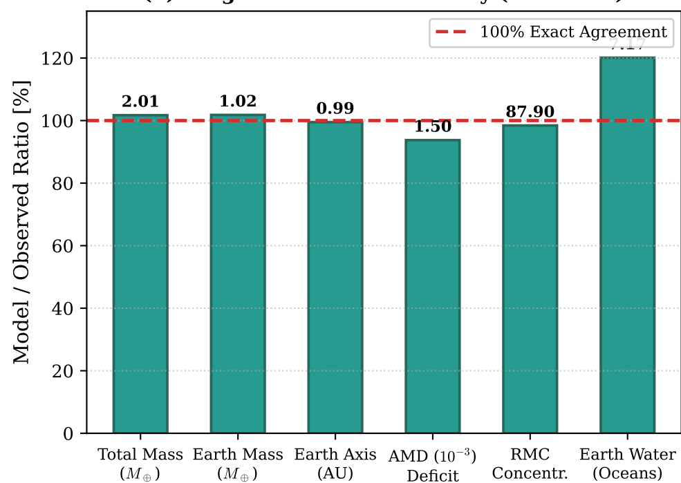
(d) Diagnostic Metrics Fidelity ( R^2 = 0.9995 )
