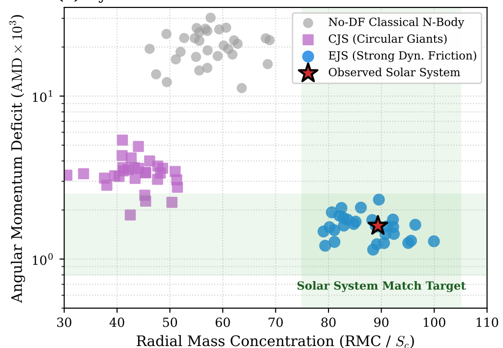
(d) Dynamical Coldness vs Radial Mass Concentration
