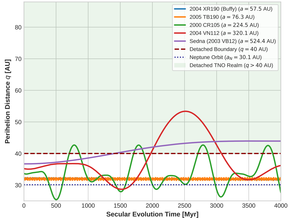
(a) Secular Perihelion Lifting Trajectories ( q(t) > 40 AU)
