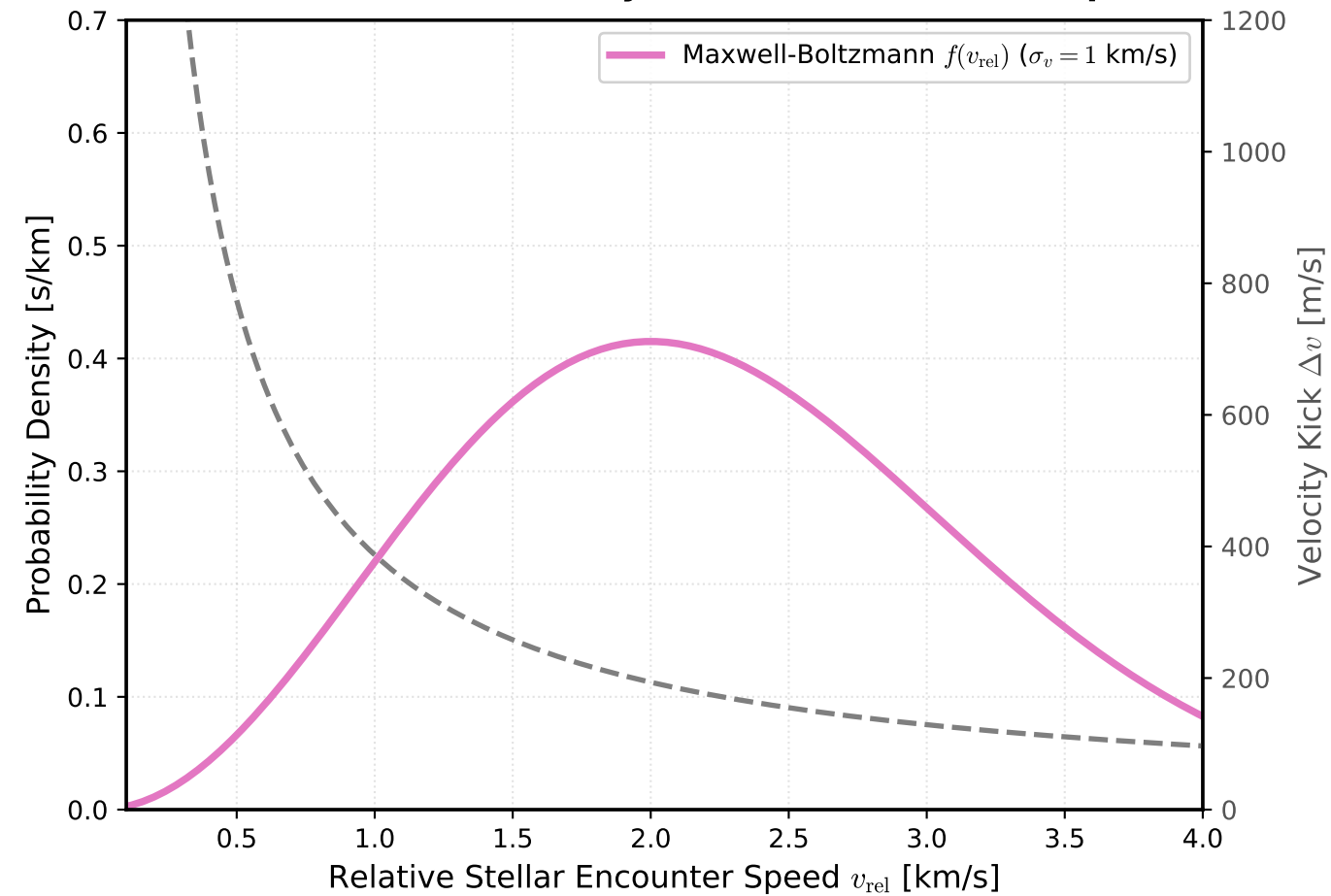
(d) Cluster Stellar Velocity Distribution & Tidal Impulse
