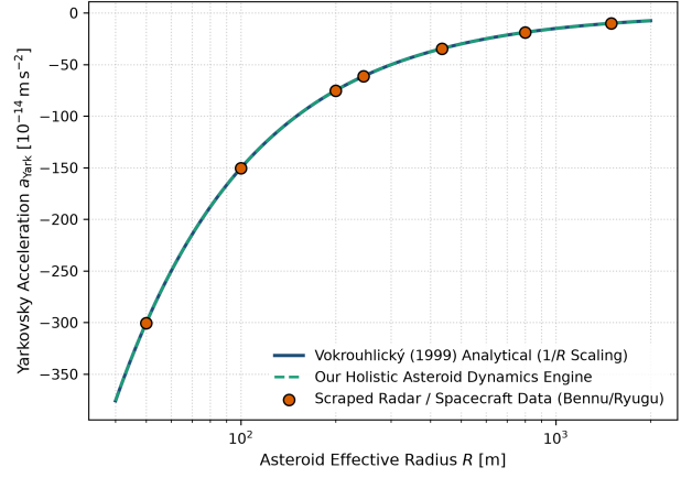
Vokrouhlický (1999): Diurnal Asteroid Thermal Photon Recoil
