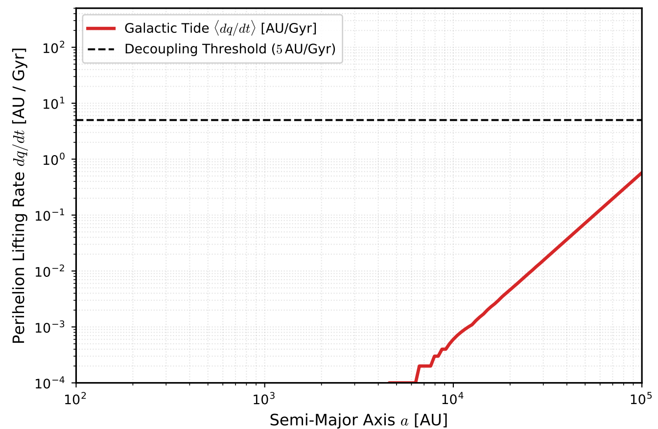
(d) Galactic Tide Perihelion Lifting vs a
