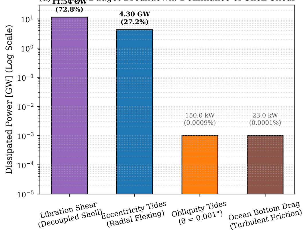
(d) Energy Budget Breakdown: Dominance of Shell Shear
