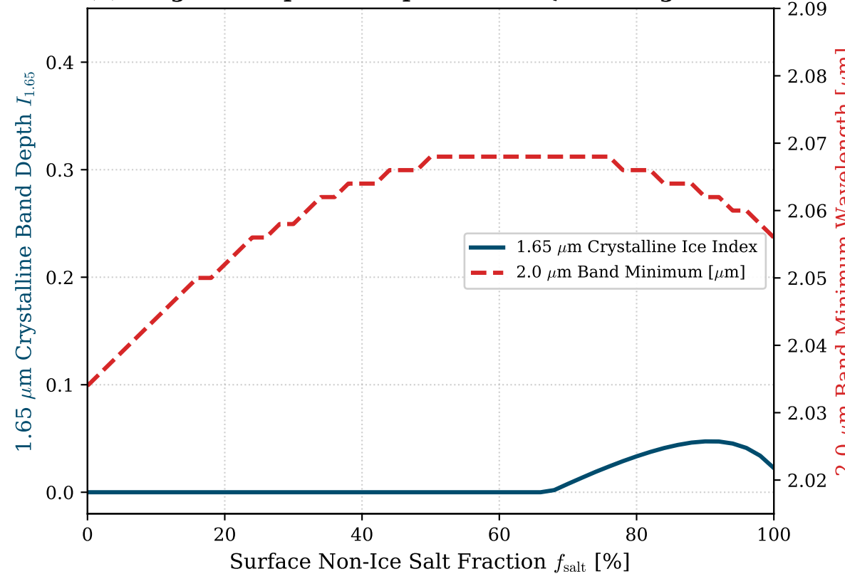
(d) Diagnostic Spectroscopic Shift & Quenching Metrics
