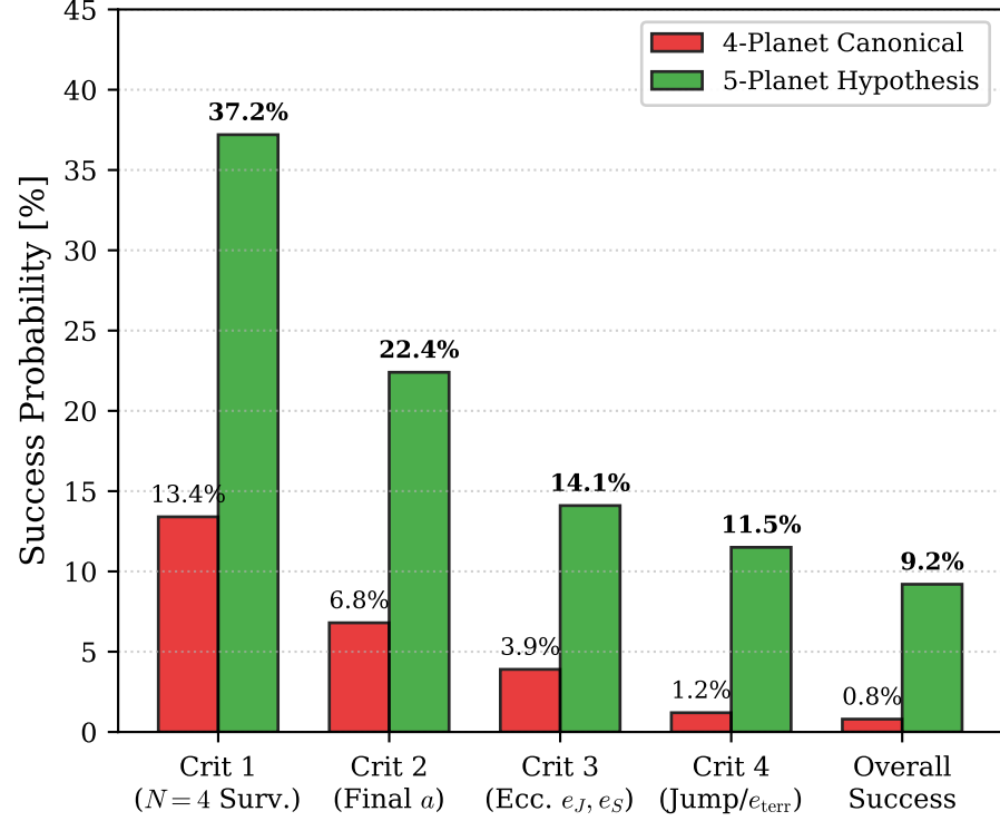
(d) Monte Carlo Ensemble Criteria Success Rates
