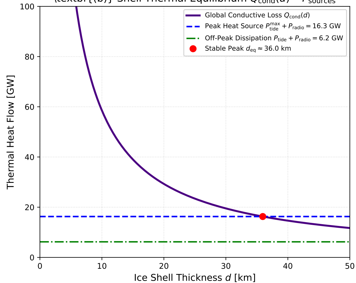
(b) Shell Thermal Equilibrium Q_{\text{cond}}(d) = P_{\text{sources}}
