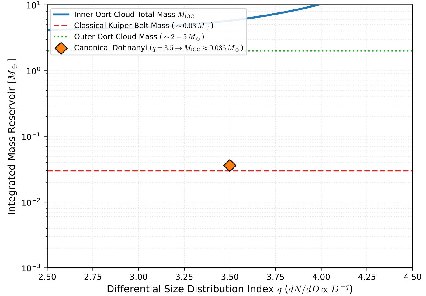
(d) Inner Oort Cloud Reservoir Mass vs Size Index q
