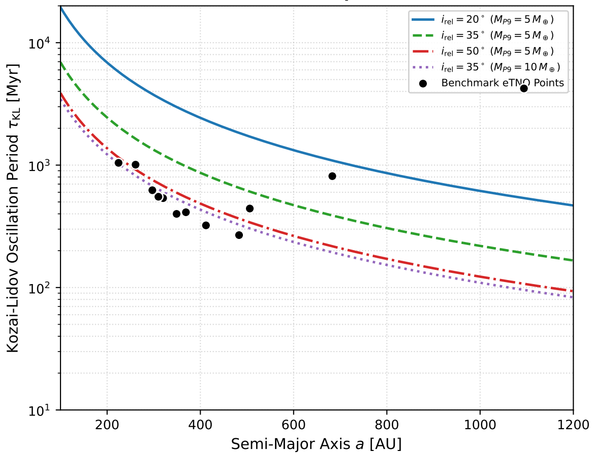
(d) Secular Timescale \tau_{\text{KL}}(a, i_{\text{rel}}) Spectrum
