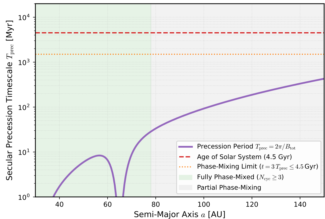
(d) Nodal Precession Timescales & Phase Mixing
