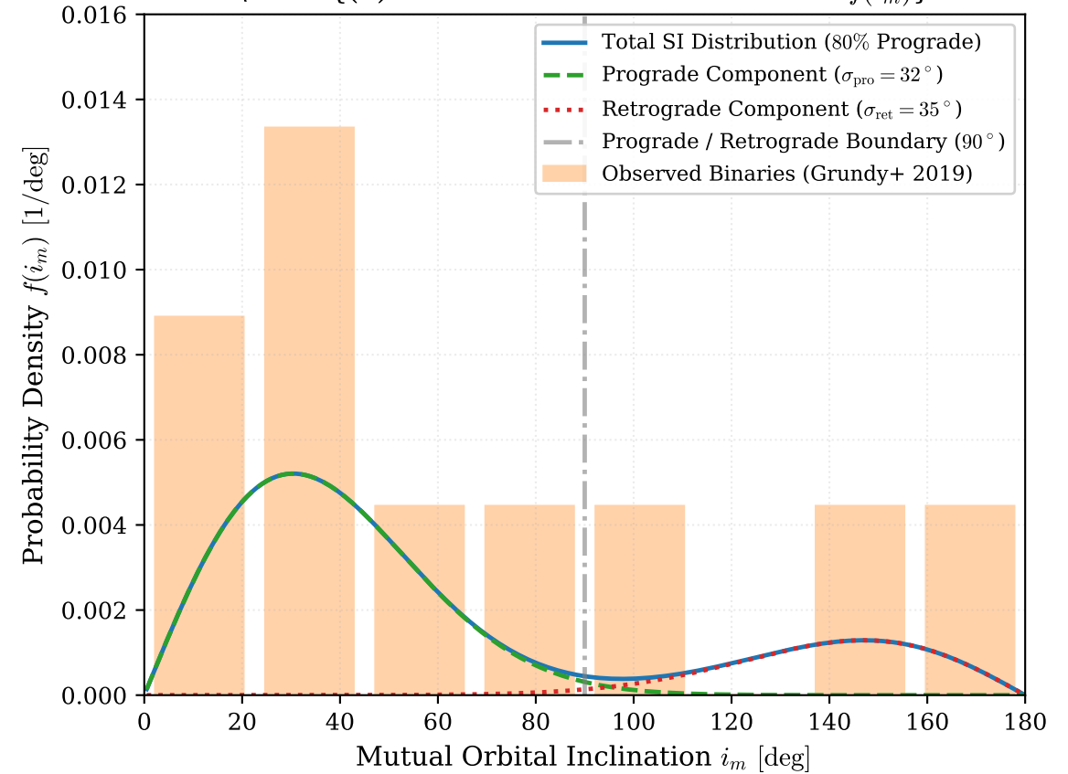
\textbf{(d) Mutual Inclination Distribution f(i_m) }
