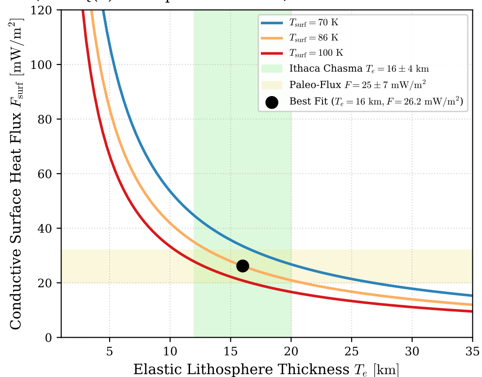
(d) Lithospheric Flexure & Inferred Paleo-Heat Flux
