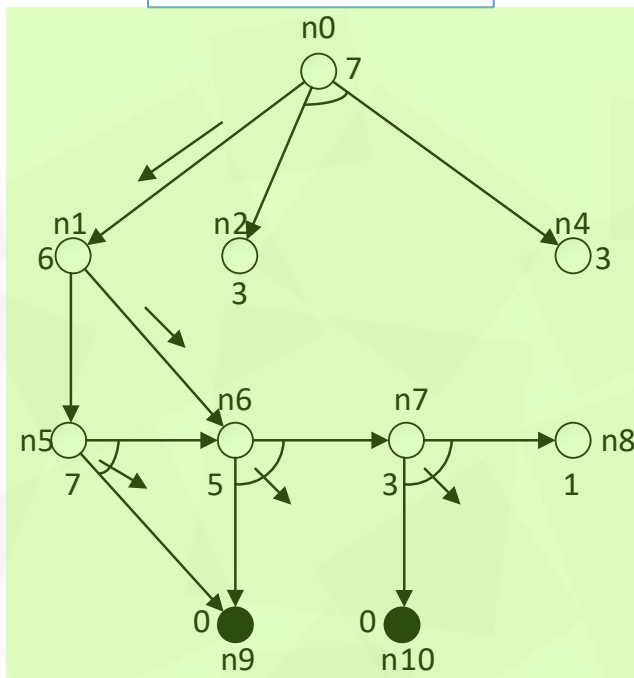
上次扩展结果 4
