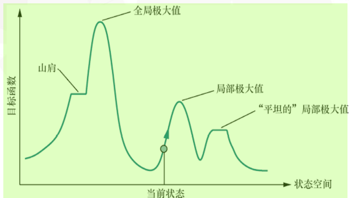
一维状态空间地形图 8
