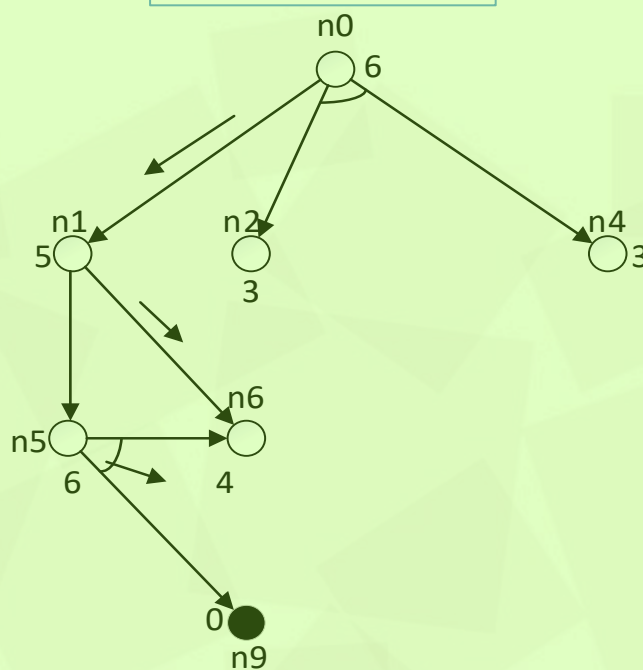
上次扩展结果 3
