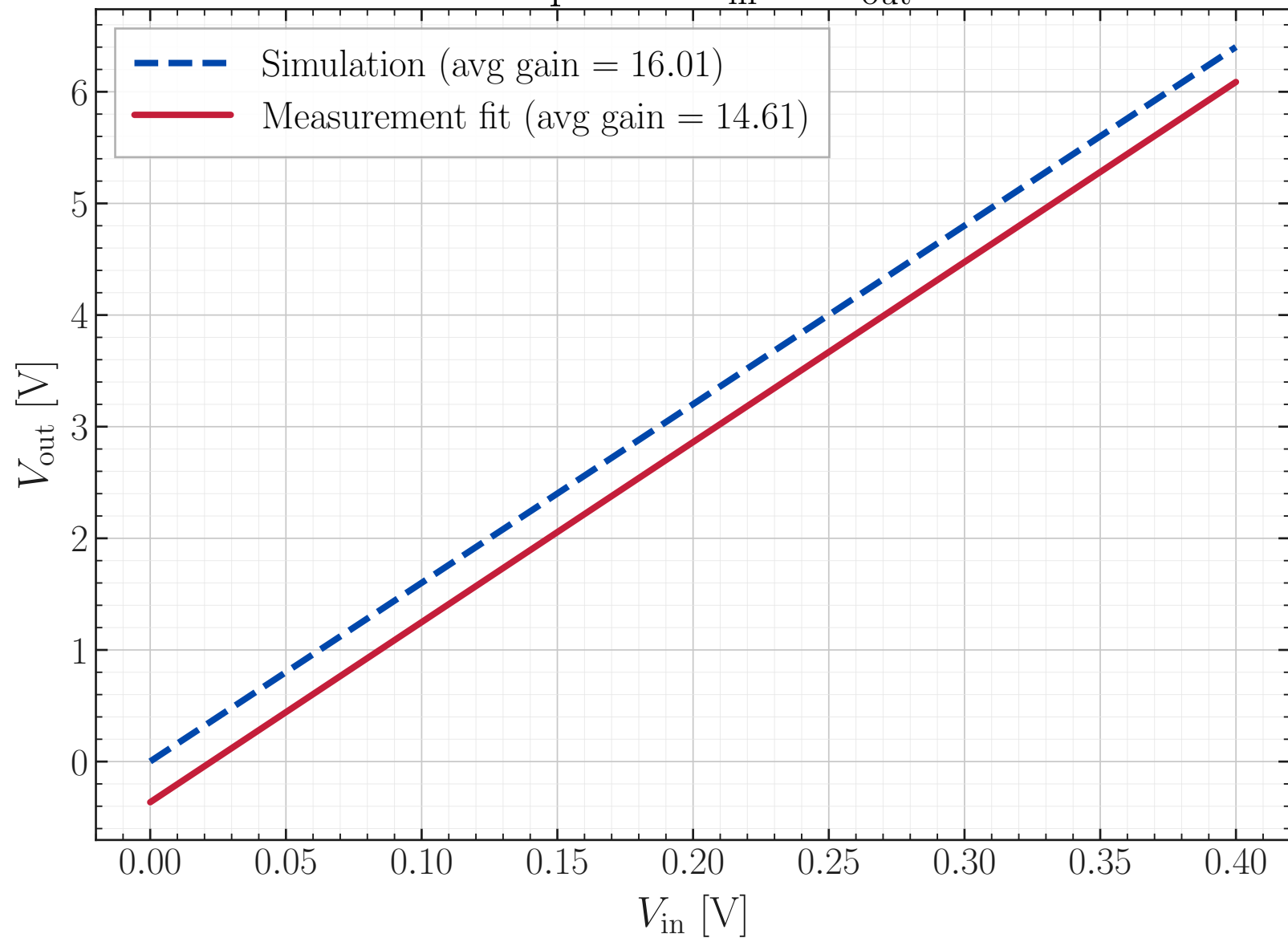
Amplifier: V_{\text{in}} vs V_{\text{out}}
