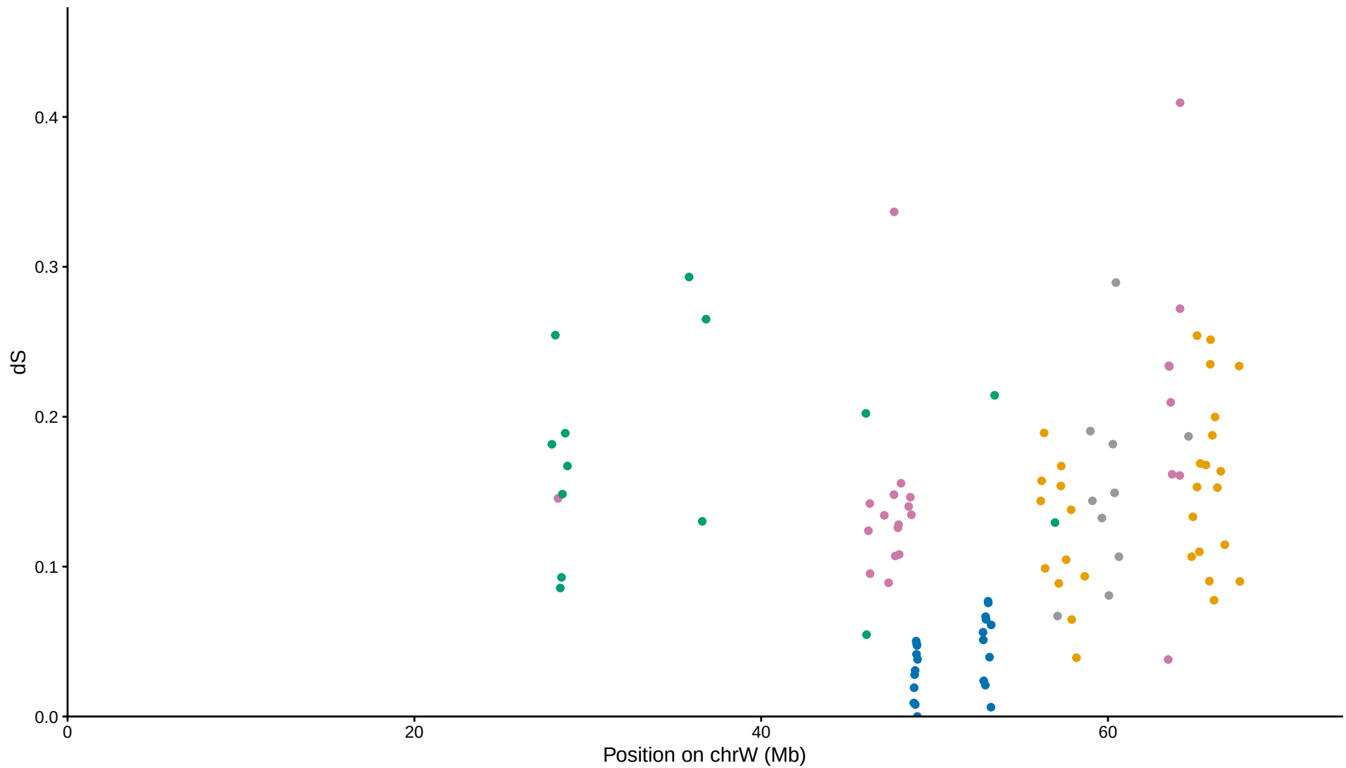
dS vs W-chromosome position (Heloderma suspectum)
