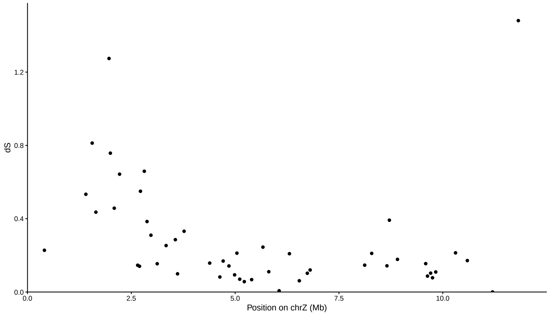
dS vs Z-chromosome position ( Varanus acanthurus )
