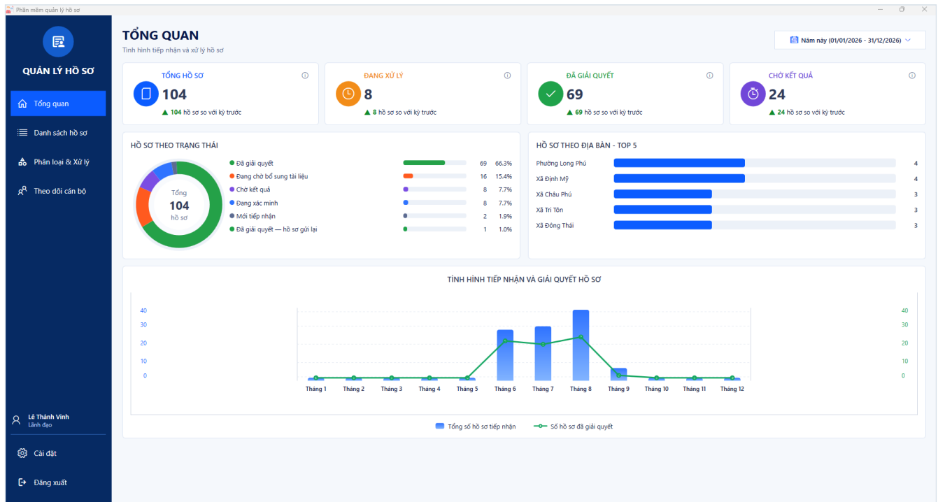
Hình 16. Trang Tổng quan
