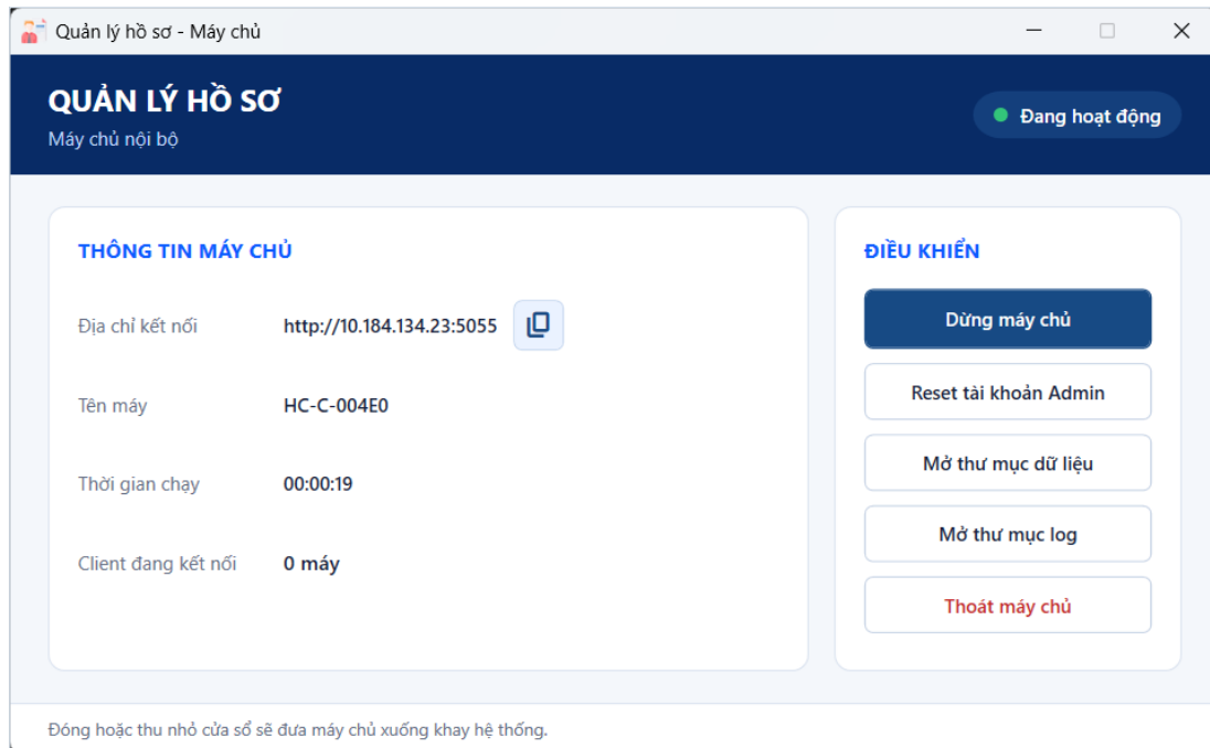
Hình 06. Bảng điều khiển QuanLyHoSo Server
