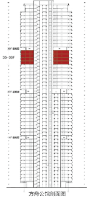
方舟公馆剖面图
