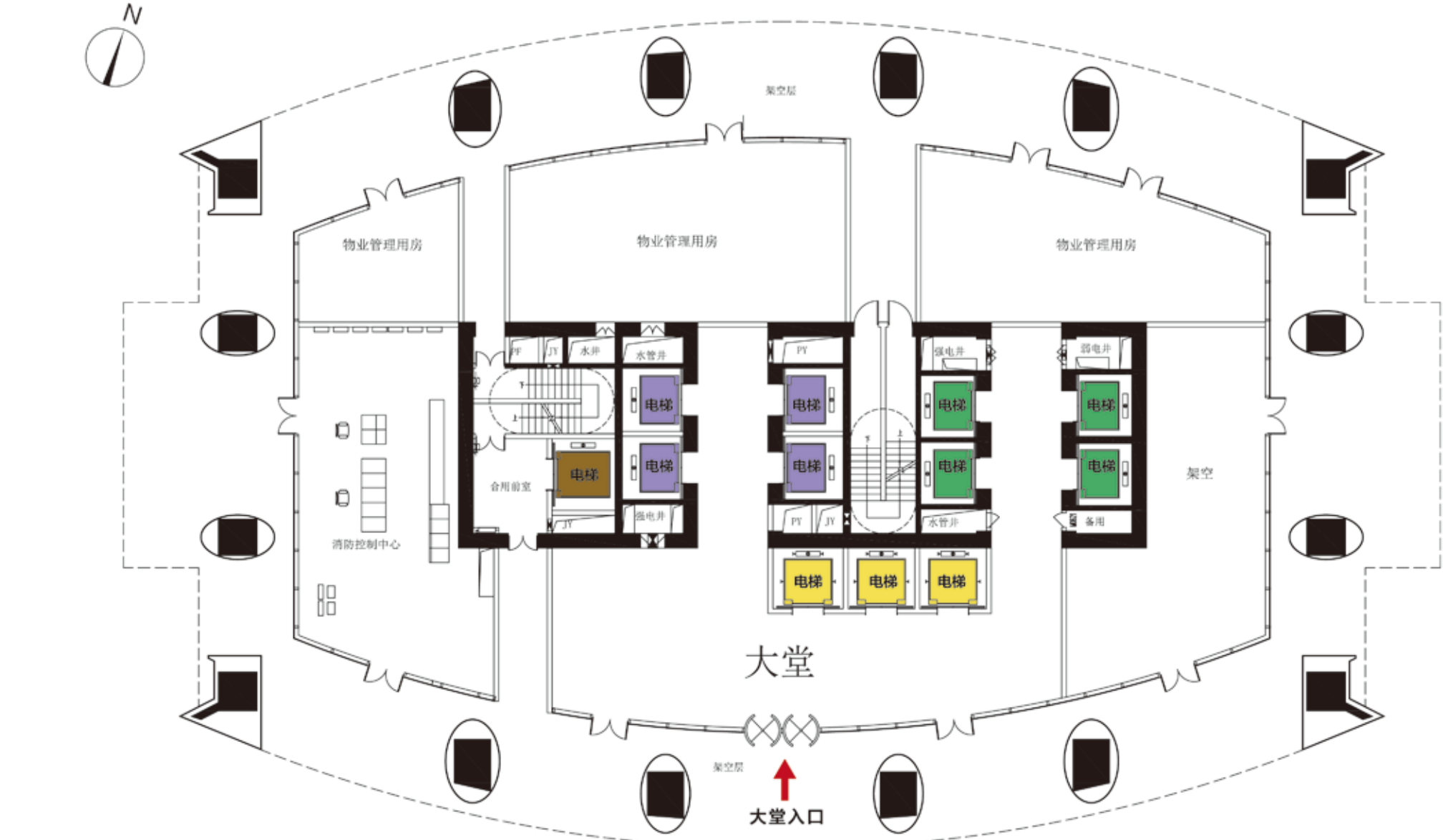
方舟公馆一层平面图
