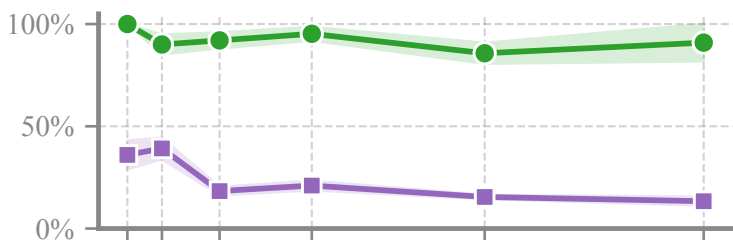
GPT-5
