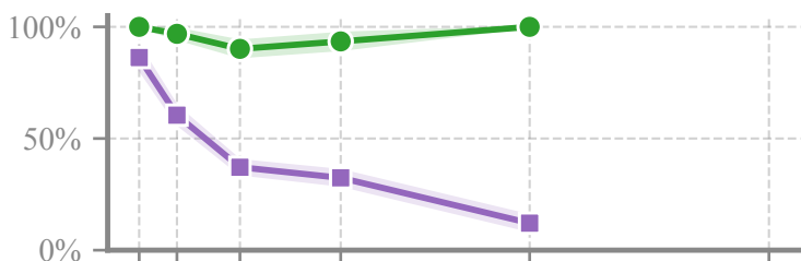
GPT-5.4
