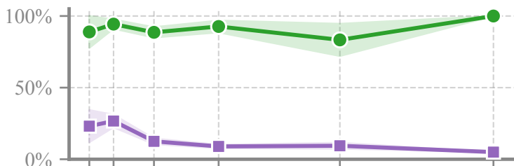
GPT-5.3 Codex
