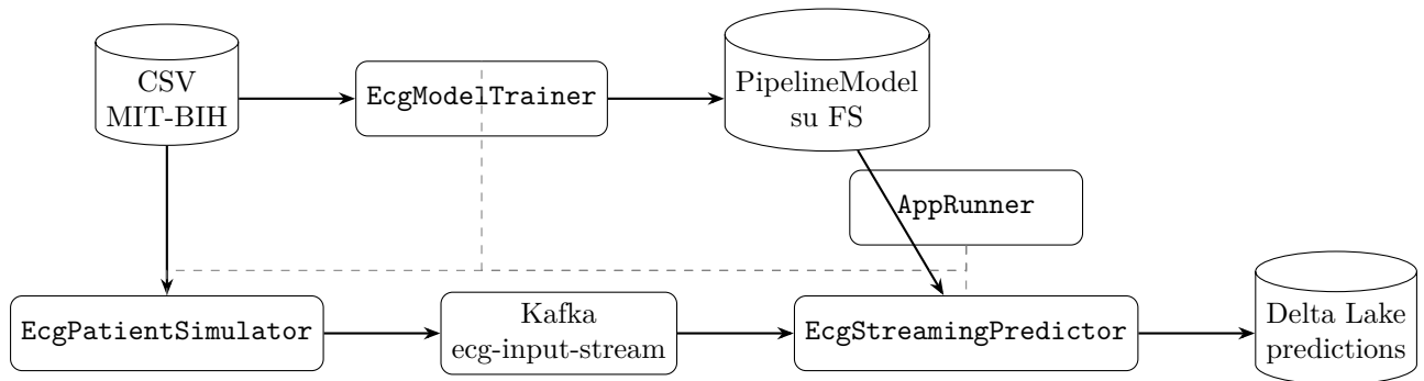
Figura 4.2: Flusso logico: training batch, ingestion simulata e inferenza streaming. Linee tratteggiate: orchestrazione AppRunner .
