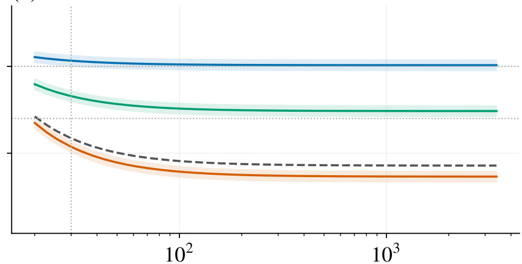
(d) GN-z11
