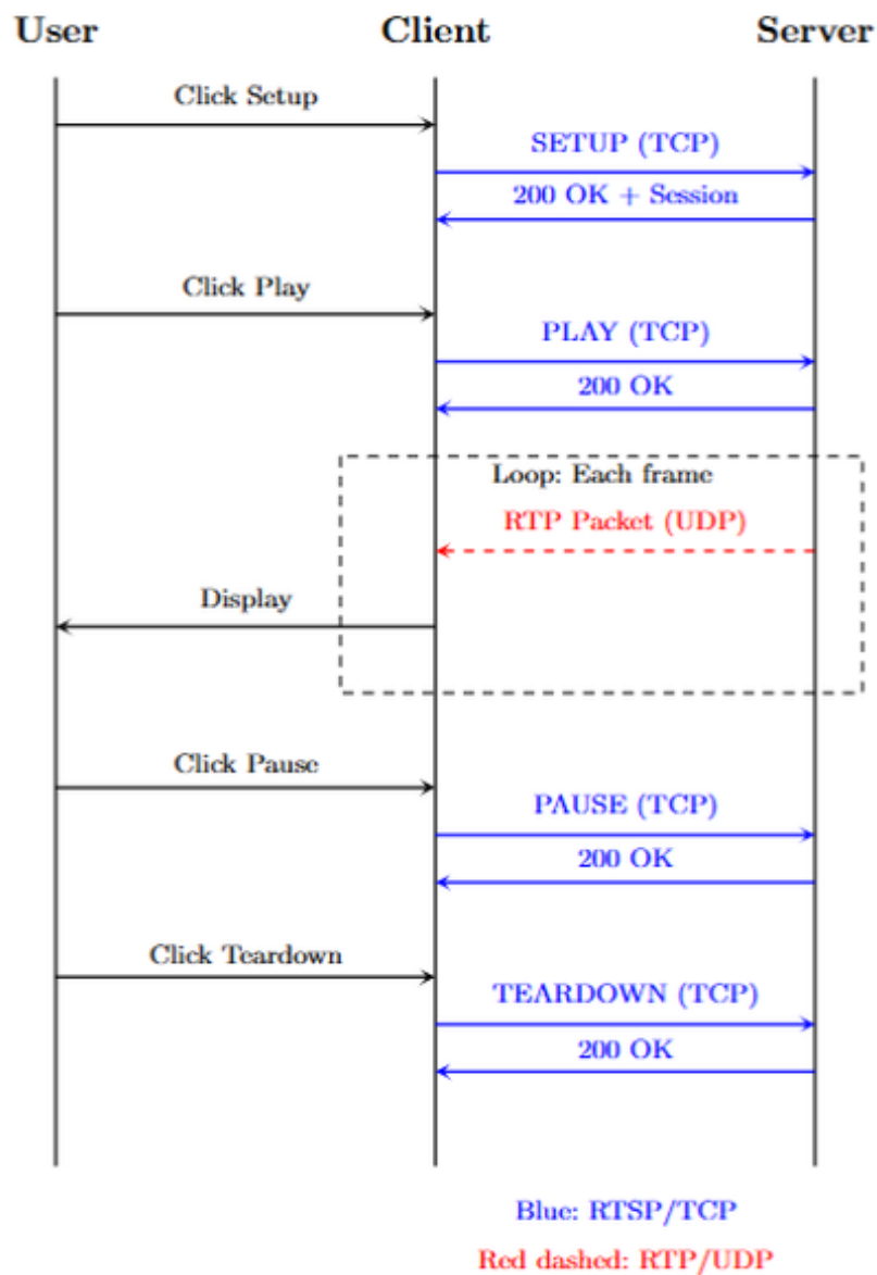
Hình 3: Sơ đồ tương tác RTSP/RTP giữa Client và Server
