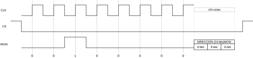
SECTOR ERASE — Opcode 0x20 (0010 0000) + Dirección (24 bits)
