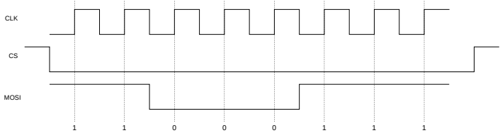
CHIP ERASE — Opcode 0xC7 (1100 0111)
