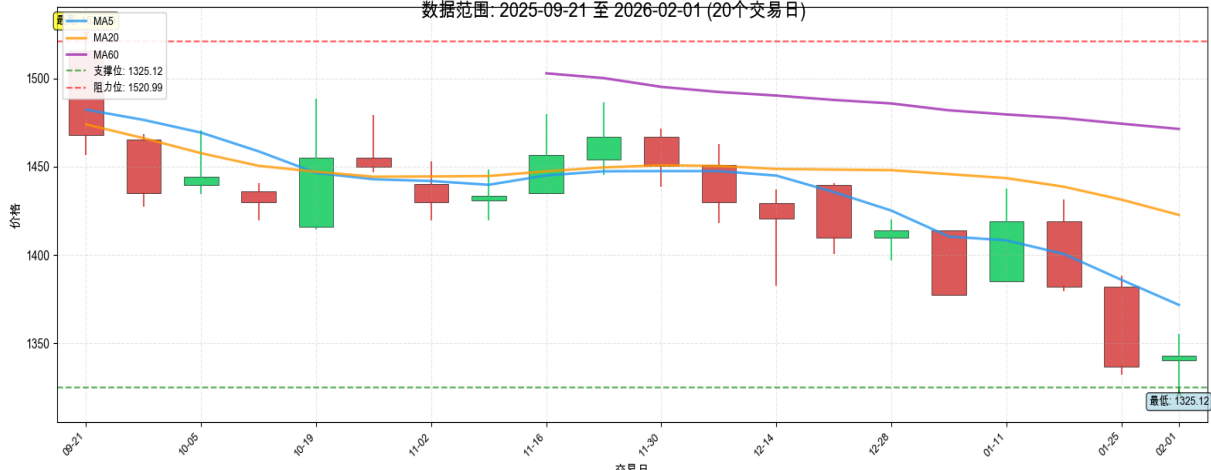
A股60099515K线图表与技术指标线 数据范围: 2025-09-21 至 2026-02-01 (20个交易日)
