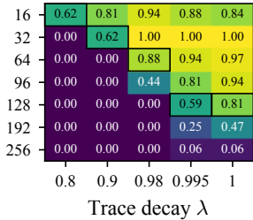
TBPTT(1)
