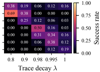
RTRL – TBPTT(1)
