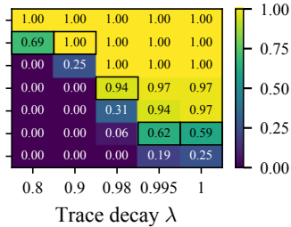
RTRL
