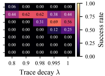
RTRL - TBPTT(1)
