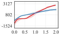
Ant
