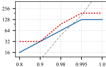
QRC( \lambda )
