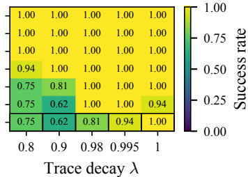
RTRL
