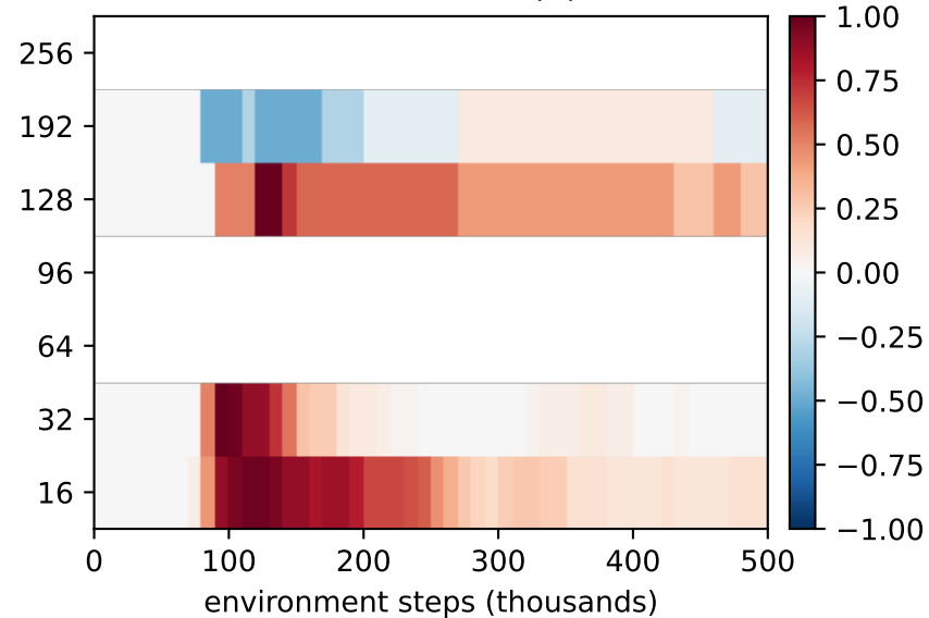
RTRL - TBPTT(1)
