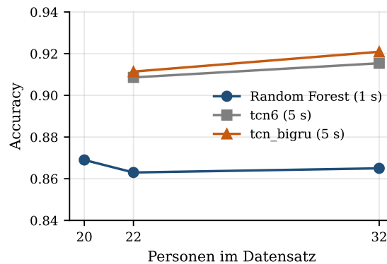
Abbildung 6: Genauigkeit in Abhängigkeit von der Zahl der Personen im Datensatz. Der Random Forest bewegt sich zwischen 20 und 32 Personen nicht, beide Netze steigen um mehr als ihre Saatenstreuung.
