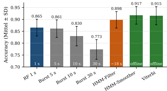
Abbildung 7: Genauigkeit derselben Random-Forest-Wahrscheinlichkeiten unter verschiedenen Dekodern (32 Personen, Mittel und Standardabweichung). Die Beschriftung am Balkenfuß gibt die Entscheidungs-Latenz an. Grau: kausaler gleitender Mittelwert. Orange: kausaler HMM-Filter. Grün: rückblickende Dekoder, die die ganze Aufnahme sehen.
