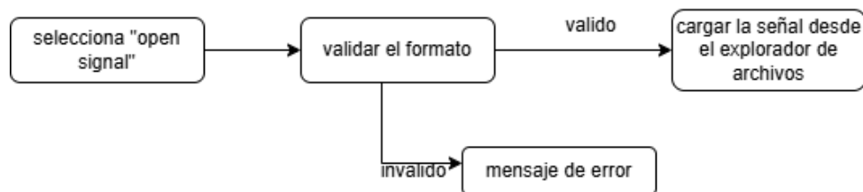
Figura 20: Flujo de carga de la señal ( Open Signal )
