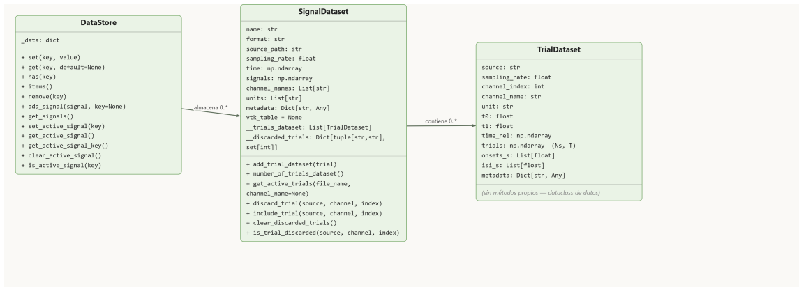
Figura 7: Diagrama de clases — componente DataStore
