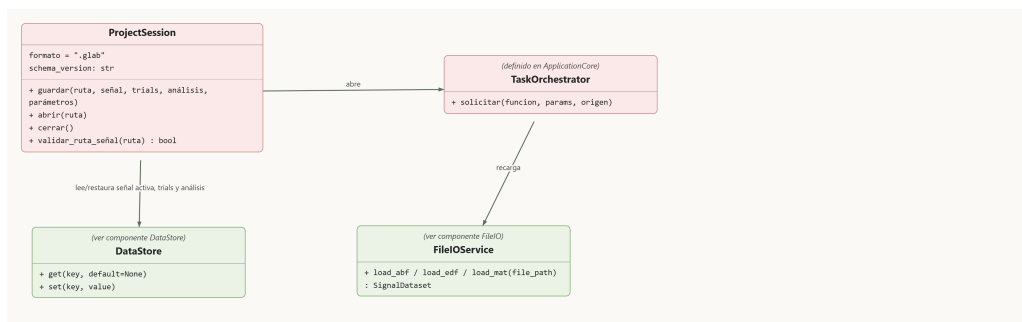
Figura 11: Diagrama de clases — componente ProjectSession
