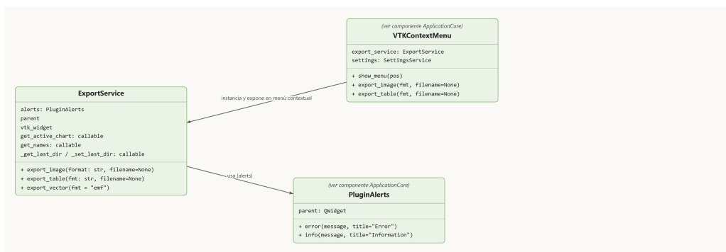
Figura 9: Diagrama de clases — componente Export
