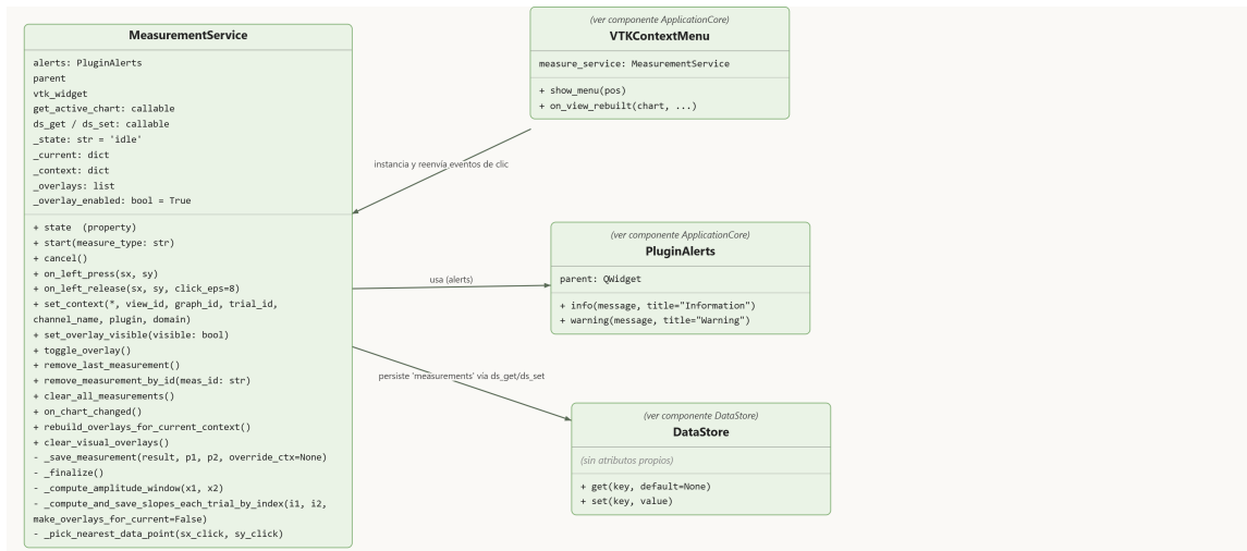
Figura 10: Diagrama de clases — componente Measurement
