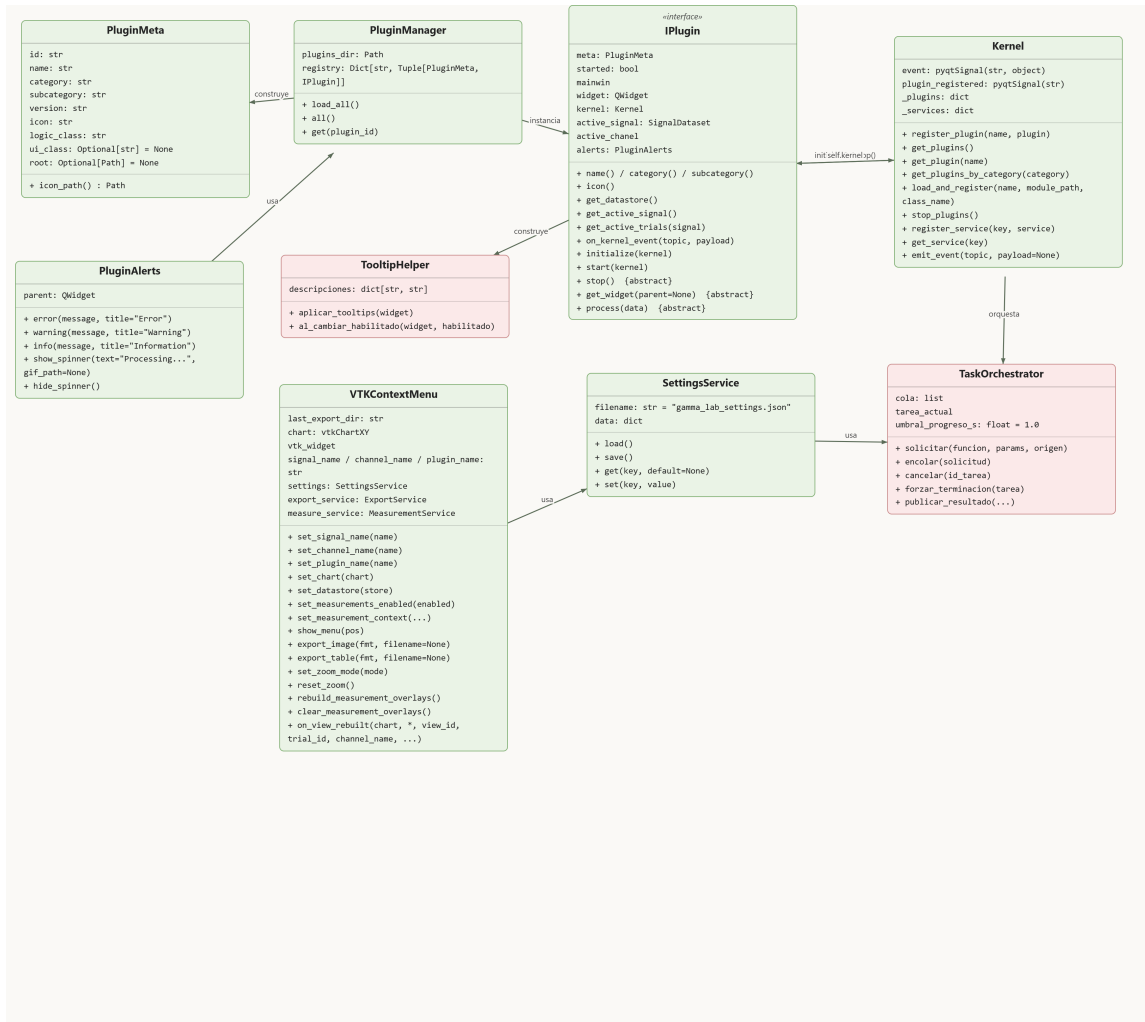
Figura 4: Diagrama de clases — componente ApplicationCore
