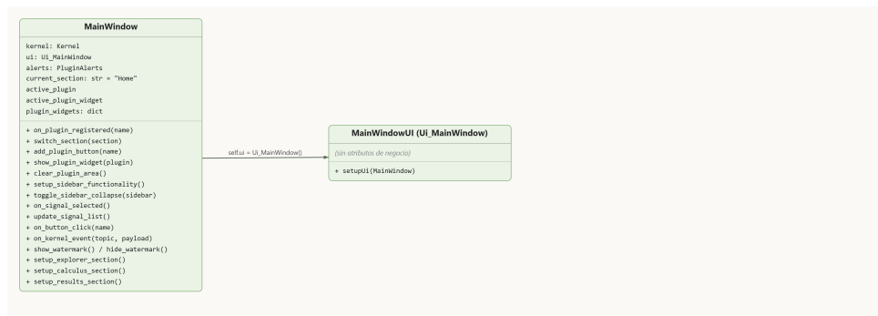
Figura 5: Diagrama de clases — componente MainUI
