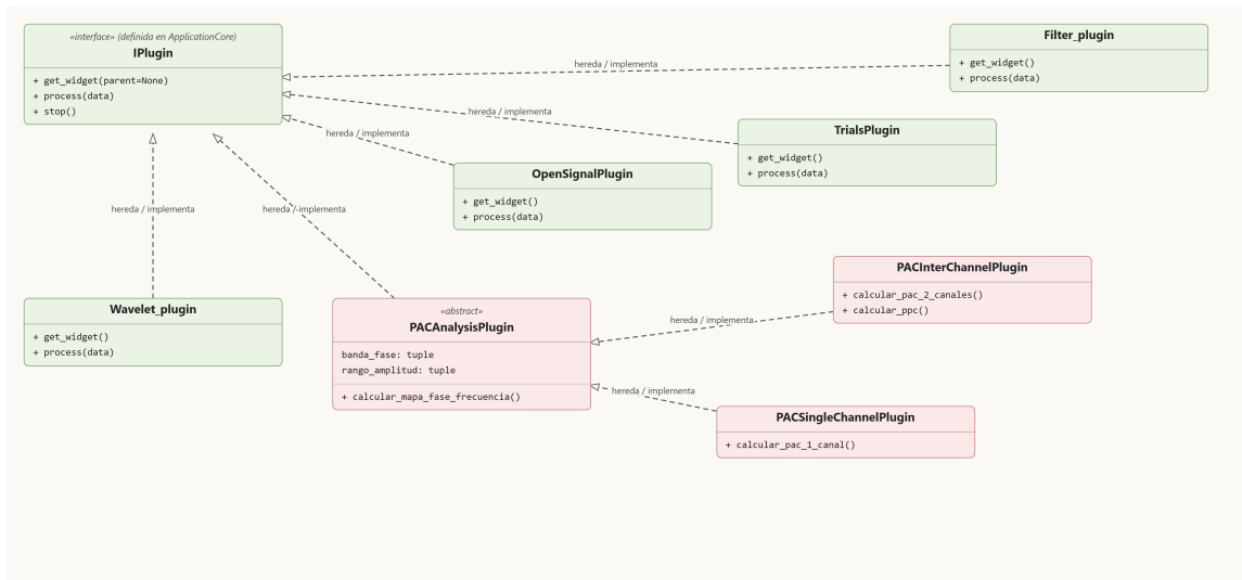
Figura 6: Diagrama de clases — componente Plugins
