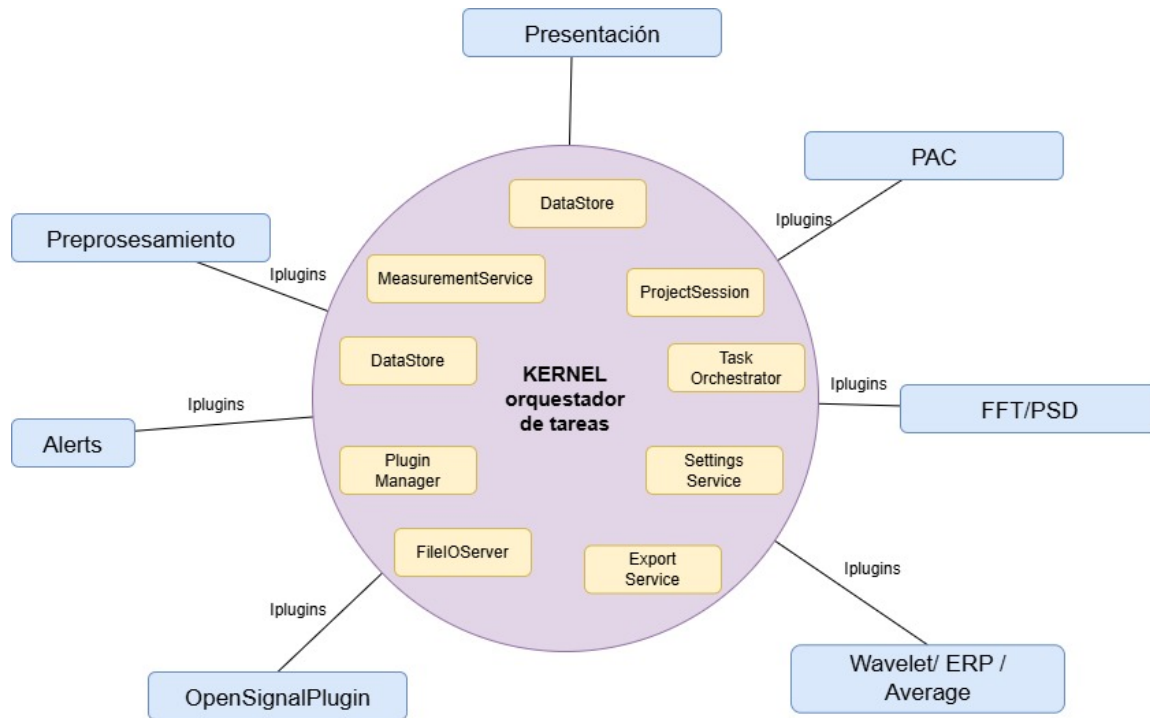
Figura 1: Diagrama conceptual de la arquitectura microkernel de GammaLab 2.0, mostrando la relación entre el núcleo central, los servicios compartidos y los plugins especializados.
