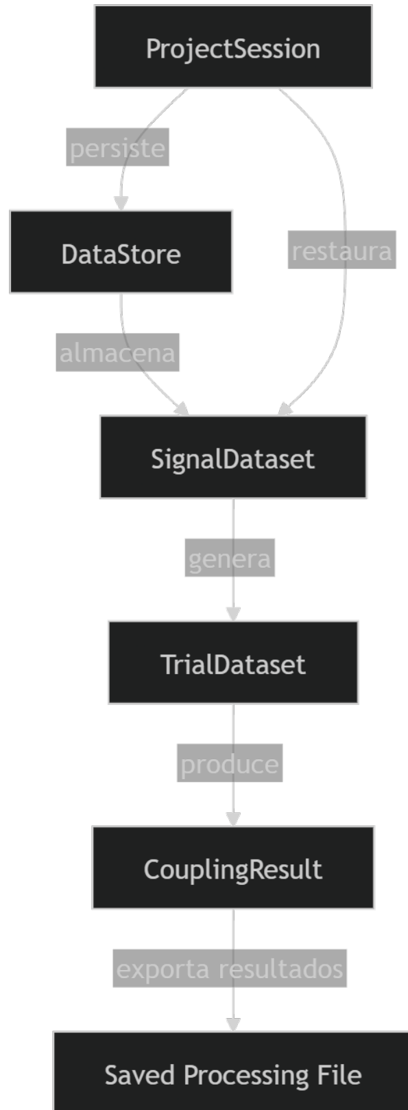
Figura 1: Modelo conceptual del dominio de Gamma Lab 2.0. Las entidades representan los componentes centrales de almacenamiento, procesamiento y persistencia de datos neurofisiológicos.
