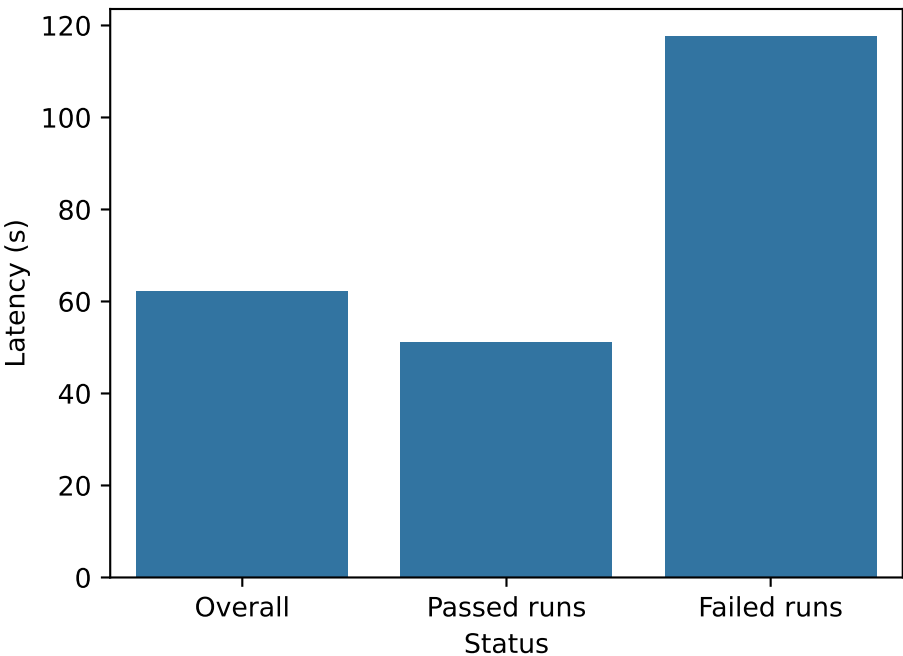
PySketch Generator
