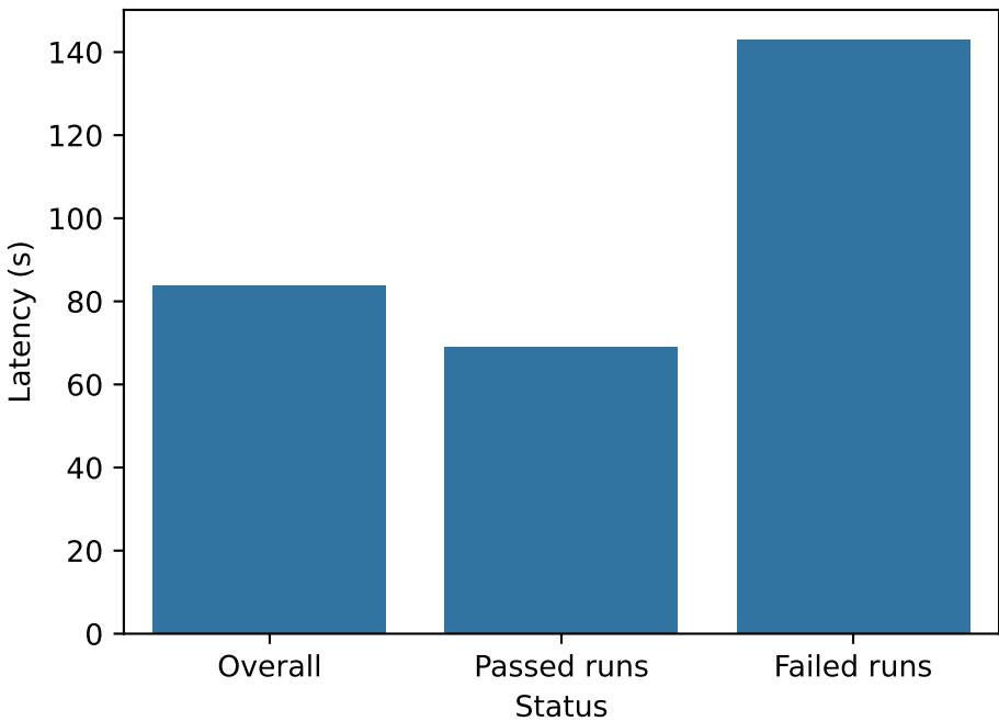
PySketch Generator
