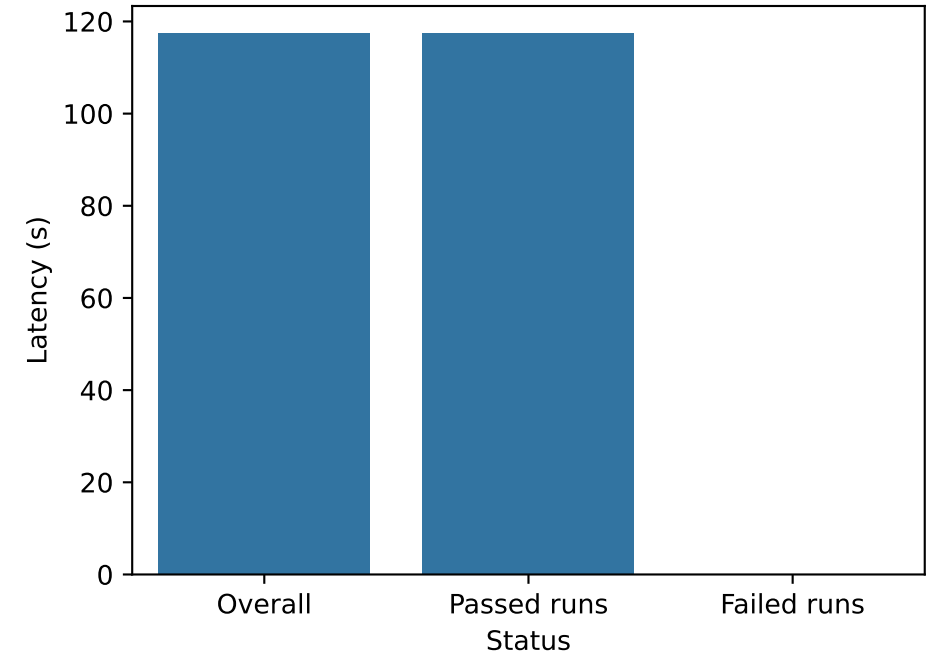
PySketch Generator
