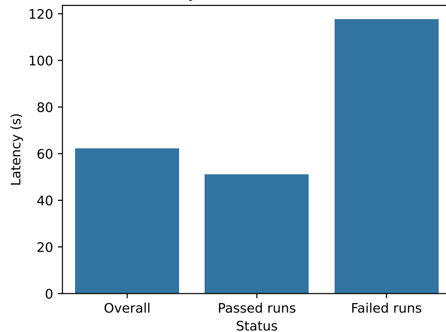
PySketch Generator
