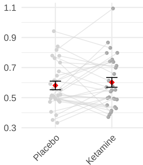
SensoryMotor
