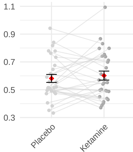
SensoryMotor
