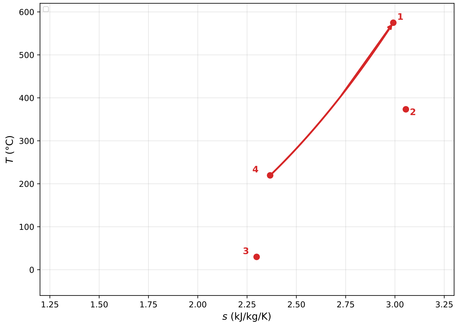
Diagramme T - s — Cycle de Brayton simple au \text{CO}_2 gazeux
