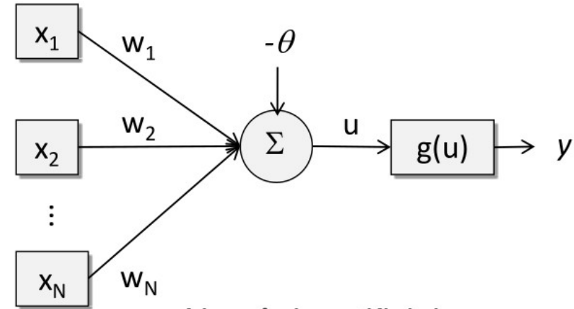
Neurônio artificial
