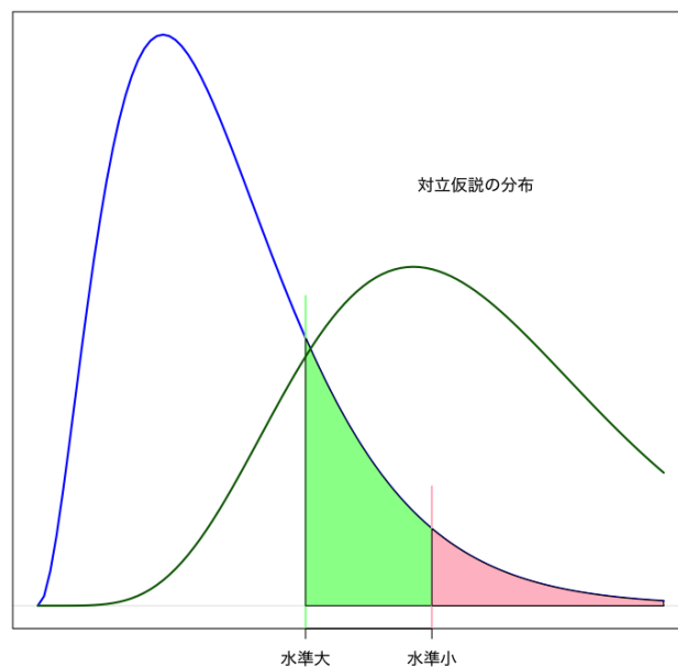
Figure 3: 検定の設計
