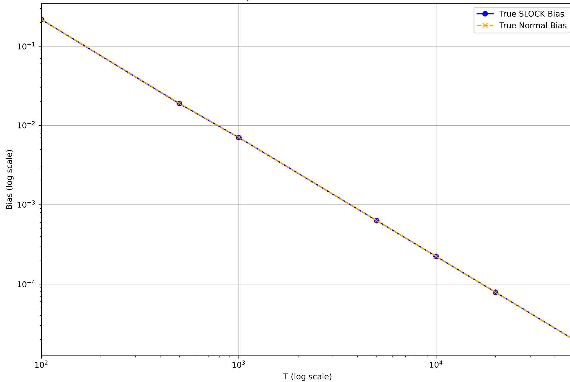
True Bias Trajectories (SLOCK vs Normal) eta=0.01
