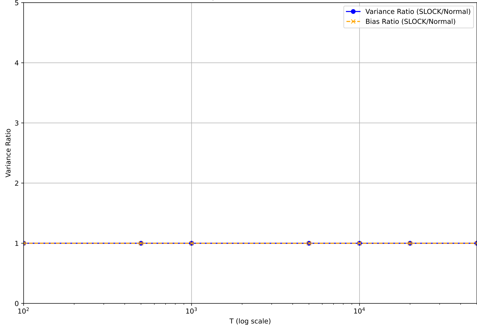
Variance Ratio Trajectories (SLOCK/Normal) eta=0.001
