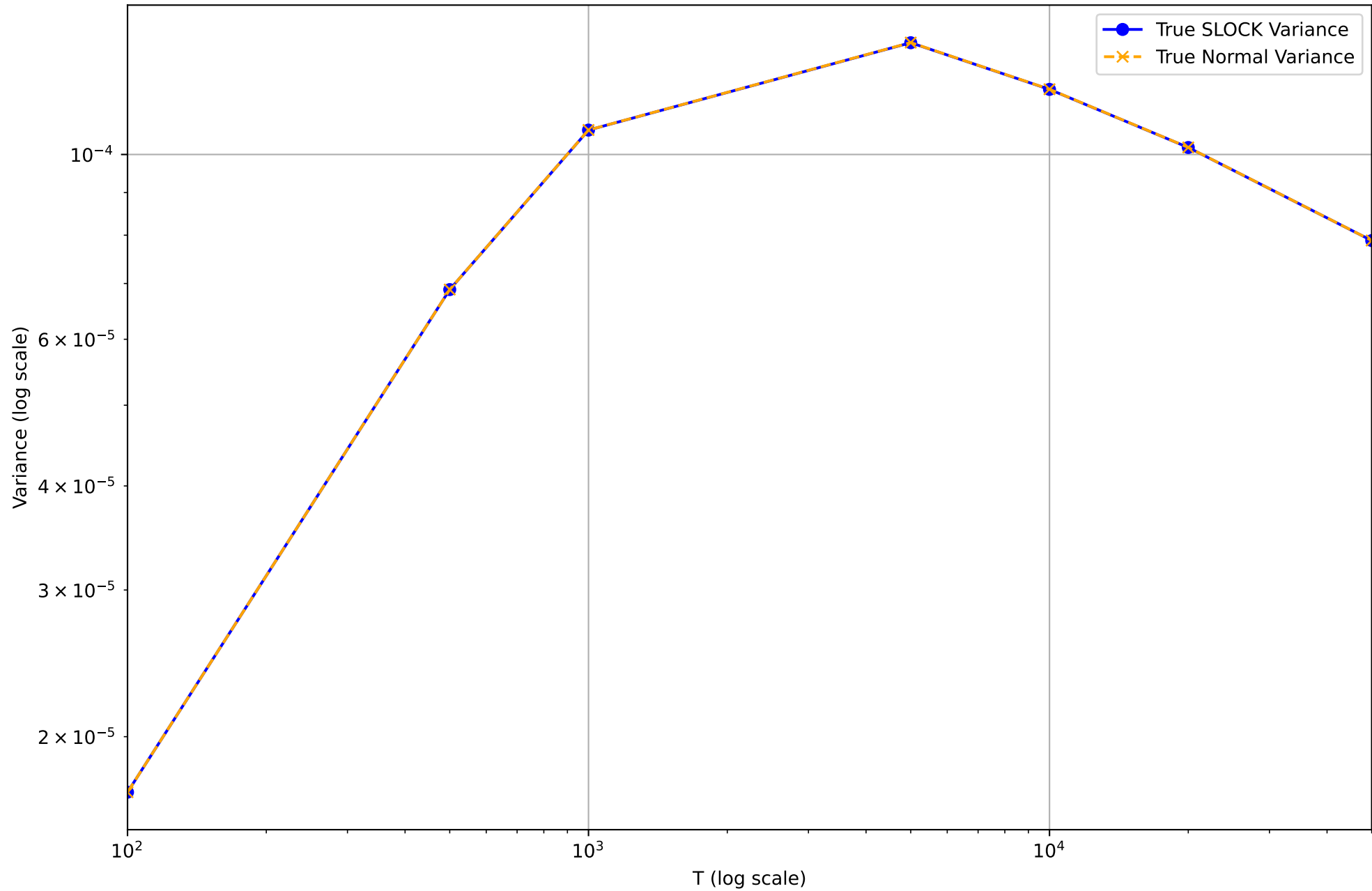
True Variance Trajectories (SLOCK vs Normal) eta=0.001
